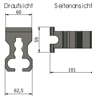
Spezial-Waffenhalter aus Vollgummi mit hohem Kautschukanteil
