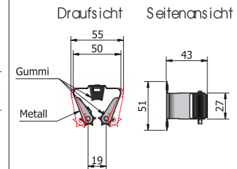
Klemmhalter aus Metall mit Gummeinsätzen
