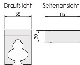
Schaumstoff-Waffenhalter 65mm Breite u.a. für doppeläufige Waffen geeignet auf Wunsch gg. Mehrpreis (die Anzahl der möglichen Waffen- halter verringert sich dadurch)
