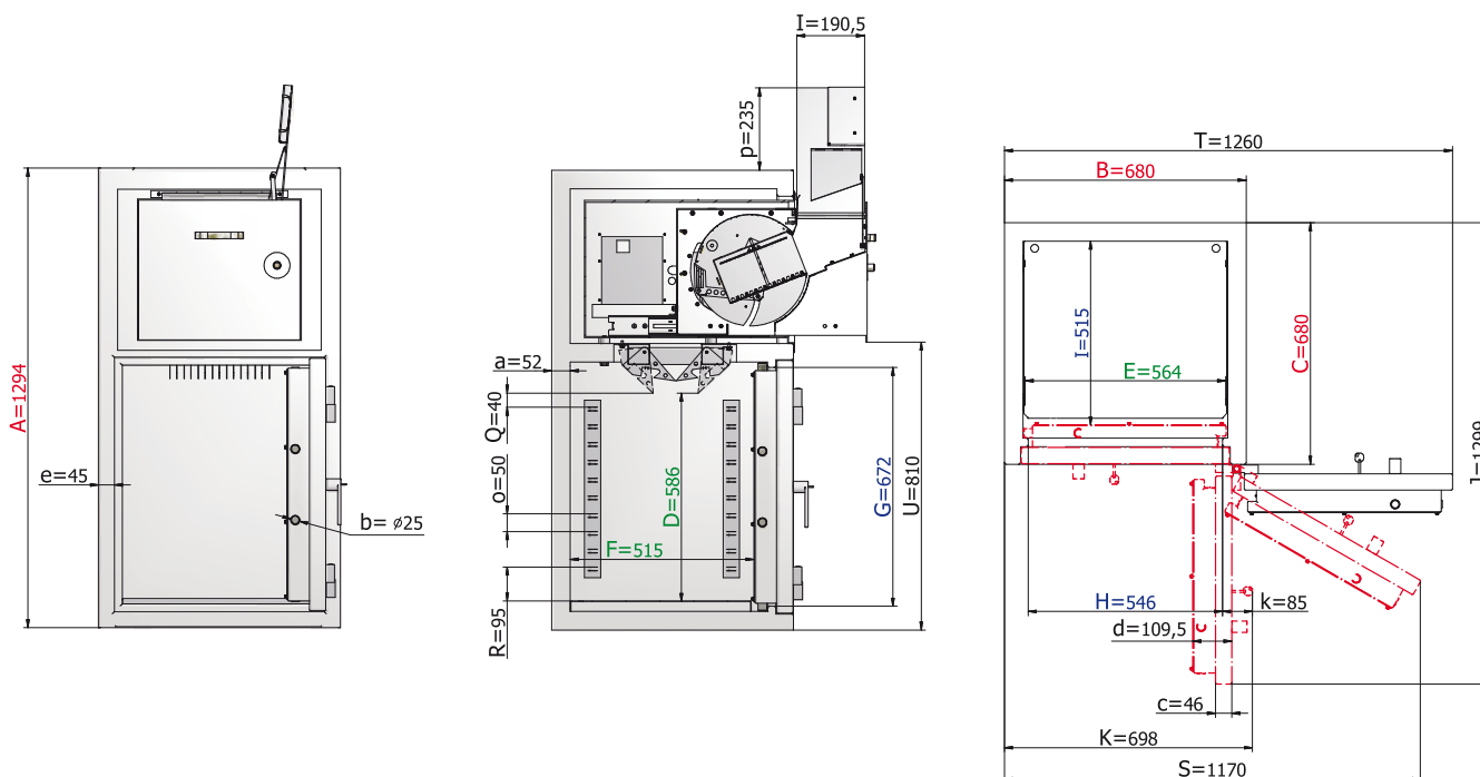
Frontansicht
