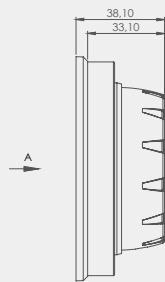
Seitenansicht
