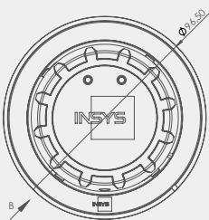
Draufsicht
