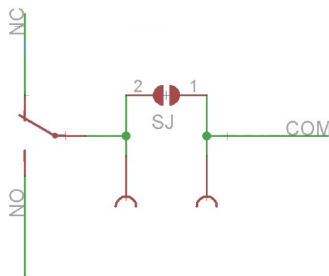
VII interne Beschaltung Ausgang
