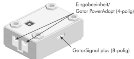
7.6.4 Gator 6000/8000/9000
