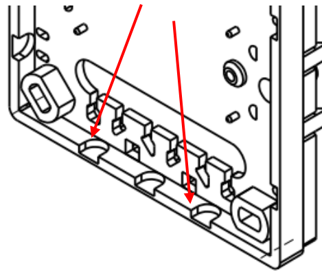
IV Leitungsausbrüche
