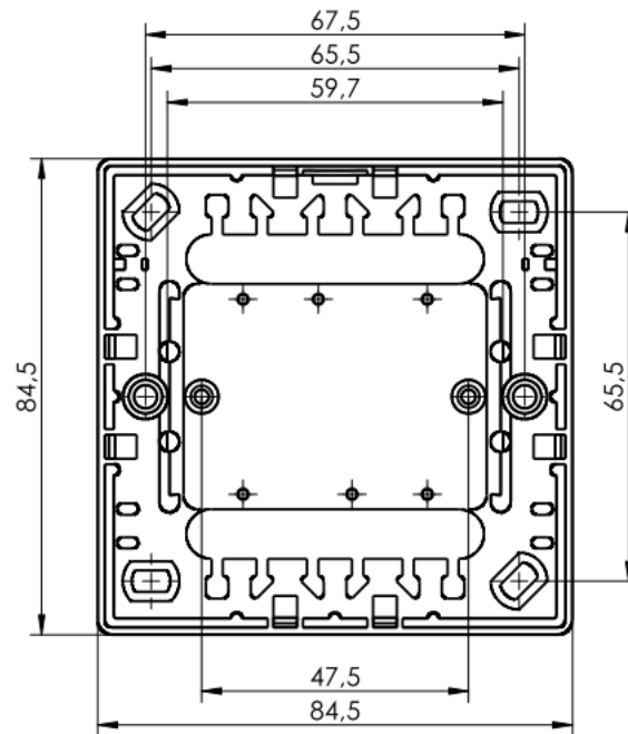
III Gehäusezeichnung
