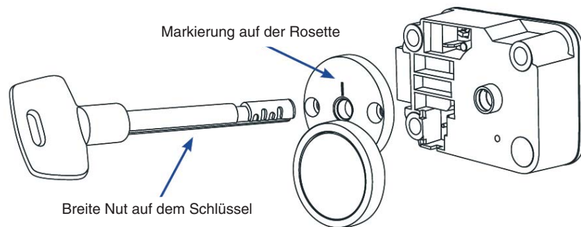
Abb. 1: Umstellbares Schlüsselschloss 2270
